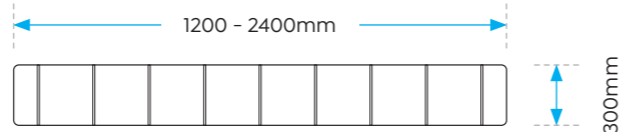
Rectangle Baffle
